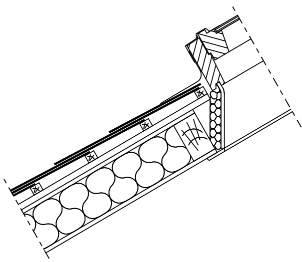
Aansluiting onderaan het dakraam
