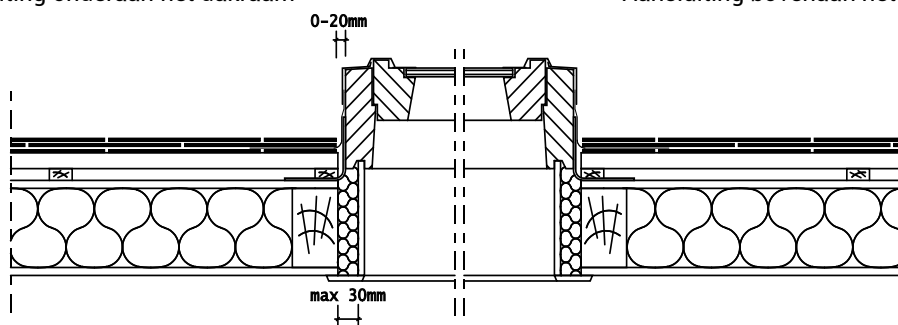
Aansluiting met de zijkant van het dakraam
