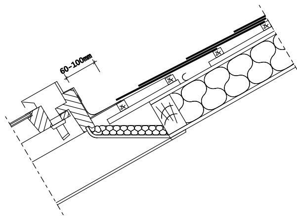
Aansluiting bovenaan het dakraam
