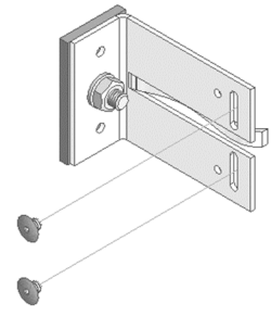
Glijdend ankerpunt
