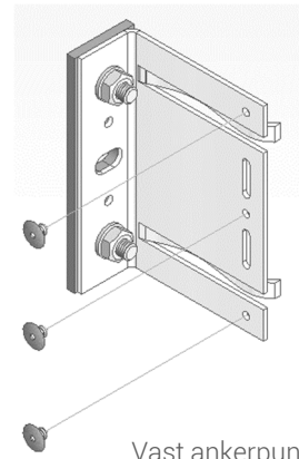
Vast ankerpunt
