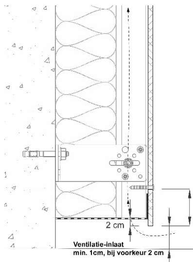
Onderzijde gevel (verticale doorsnede)
